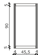
BOK
