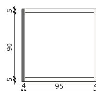
BOK
