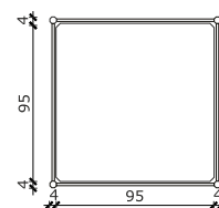
GÓRA
